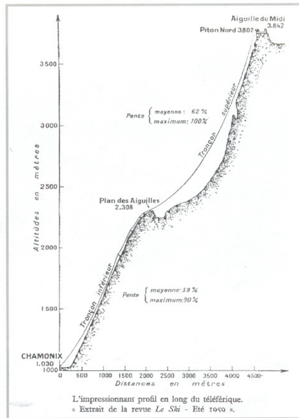
Profil en travers paroi Aiguille du Midi Cross section of the wall of the "Aiguille du Midi"
